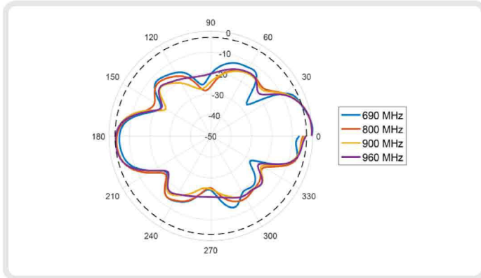
E-Plane: 690 - 960 MHz
