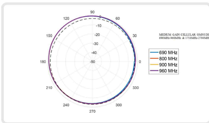
H-Plane: 690 - 960 MHz
