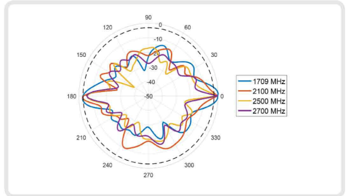
E-Plane: 1700 - 2700 MHz
