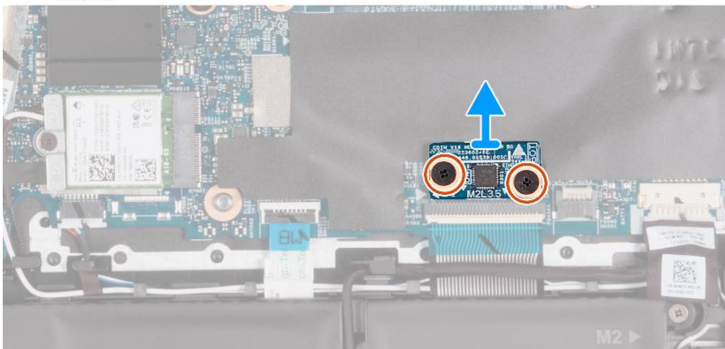
2x M2x3.5
